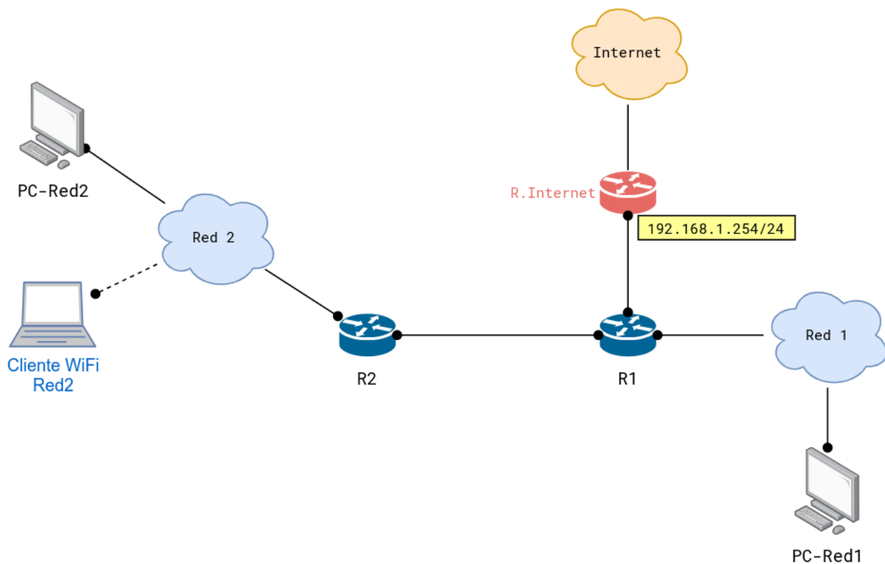
Topología Escenario 3
